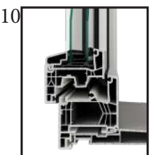
10 PERFORM76 : profil étanche grâce à ses 3 joints & 6 chambres
