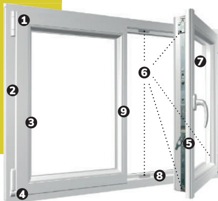
Système sécurité : rouleau champignon anti-dégondage et anti-effraction
