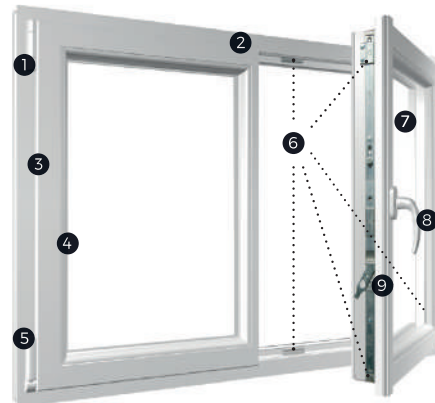
Système anti-fausse manœuvre et levier de vantail
