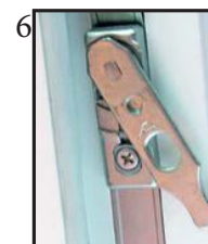
6 Système anti-fausse manœuvre et levier de vantail.
