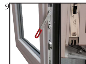
9 Compression et sécurité doublée grâce à la crémonne du semi-fixe.
