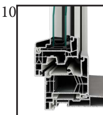
10 PERFORM76 : profil étanche grâce à ses 3 joints & 6 chambres
