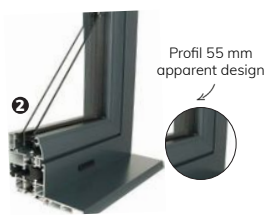
Profil 55 mm apparent droit
