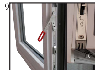
Compression et sécurité doublée grâce à la crémonne du semi-fixe.
