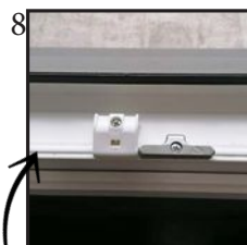
Câble anti-fatigue et jonc de finition en partie basse du dormant.
