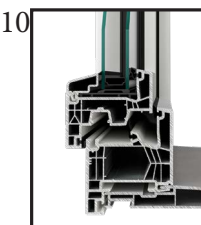
PERFORM76 : profil étanche grâce à ses 3 joints & 6 chambres
