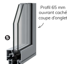
Profil 65 mm ouvrant caché coupe droite
