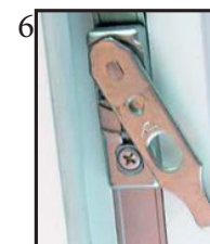
Système anti-fausse manœuvre et levier de vantail.
